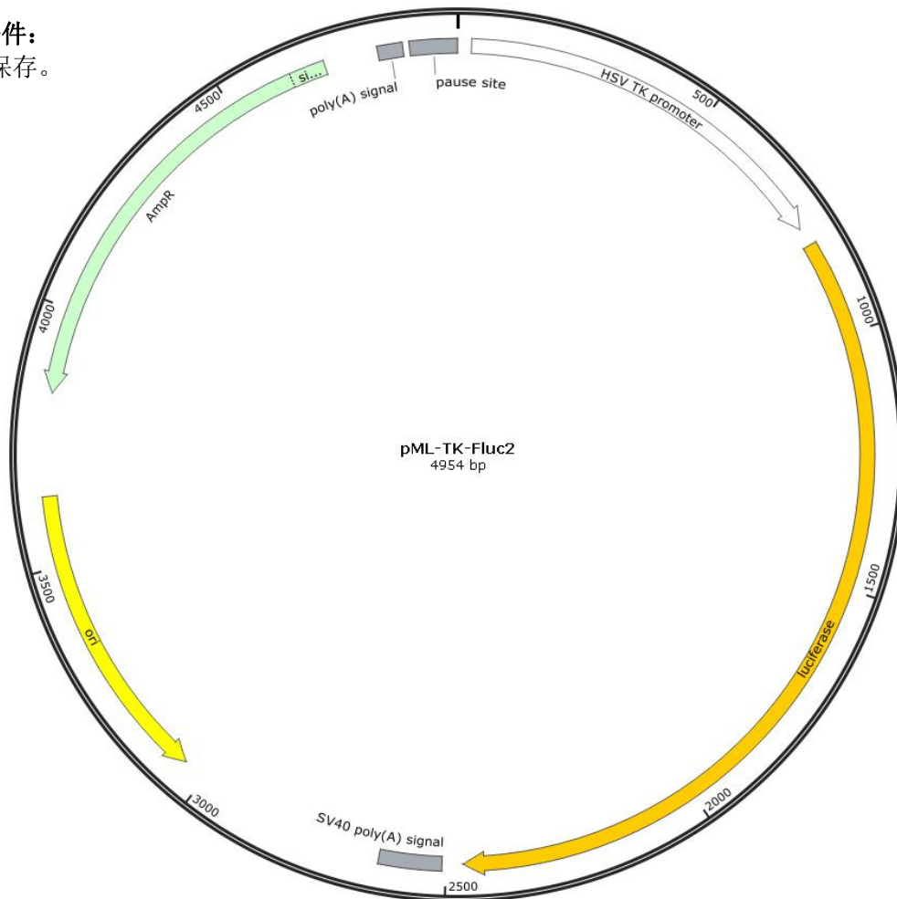
图1. pML-TK-Fluc2质粒图谱
