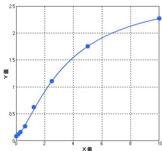
人 Prolactin 参考标准曲线
