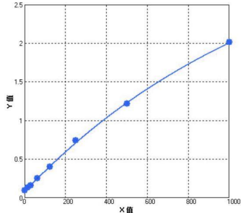
人 Tissue Factor 参考标准曲线
