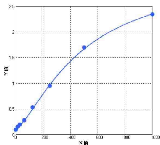
人 CD40 参考标准曲线
