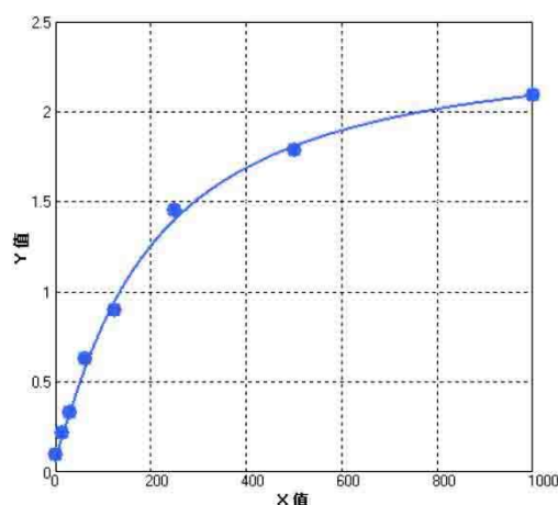
小鼠 EPO 参考标准曲线
