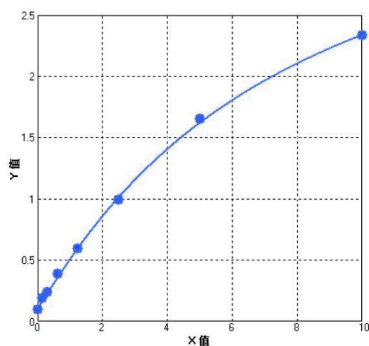
人 Enolase 2 参考标准曲线
