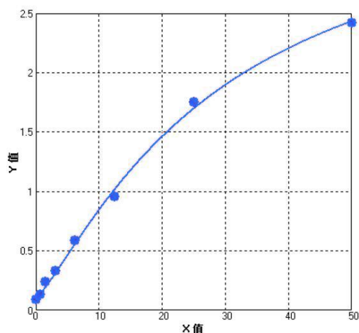
人 MGMT 参考标准曲线
