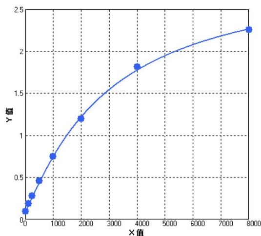
小鼠 IL-7 参考标准曲线
