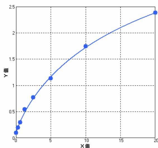
小鼠 Leptin R 参考标准曲线
