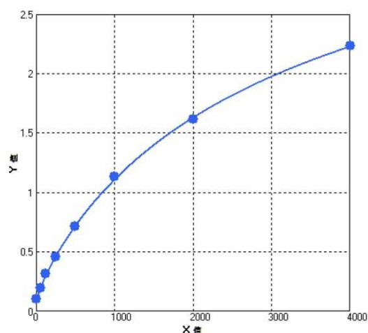
小鼠 IL-16 参考标准曲线
