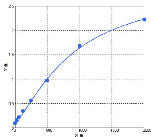
小鼠 FGF-1 参考标准曲线
