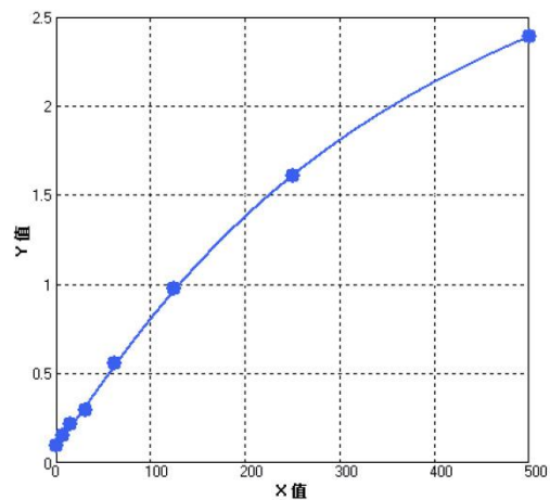
小鼠 CD47 参考标准曲线
