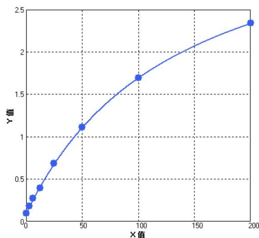
人 GSN 参考标准曲线
