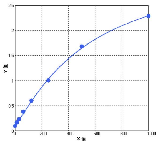
人 Granzyme A 参考标准曲线
